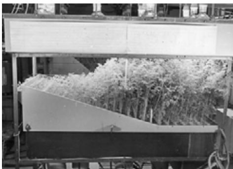
Установка «Самород», вид сбоку
